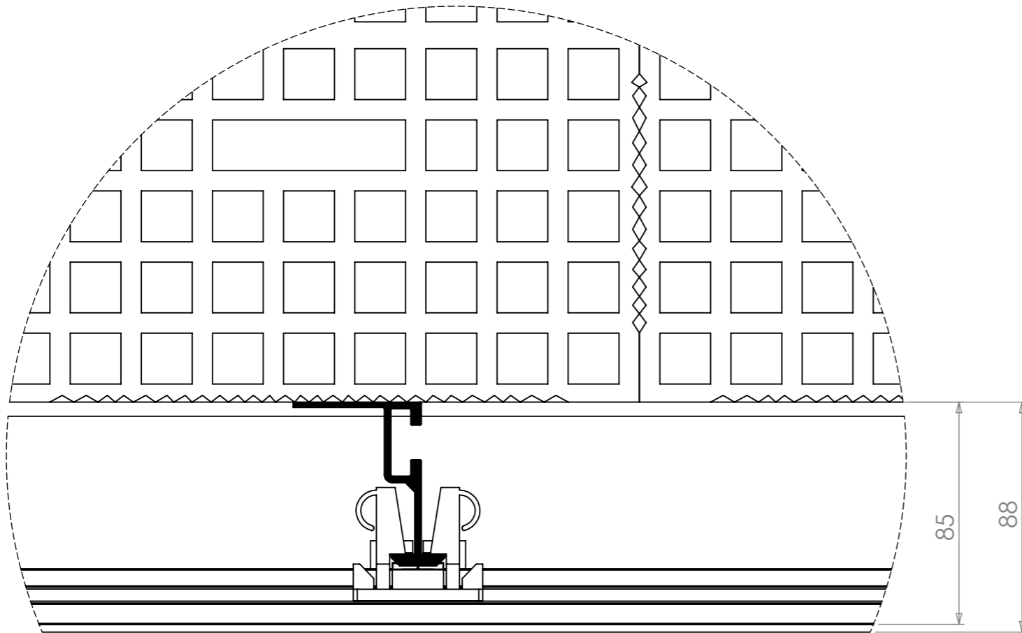
DETTAGLIO F SCALA 1 : 2
