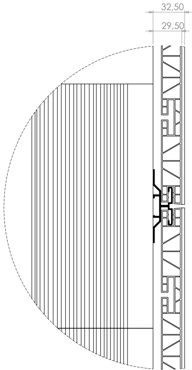
DETTAGLIO D SCALA 1:2
