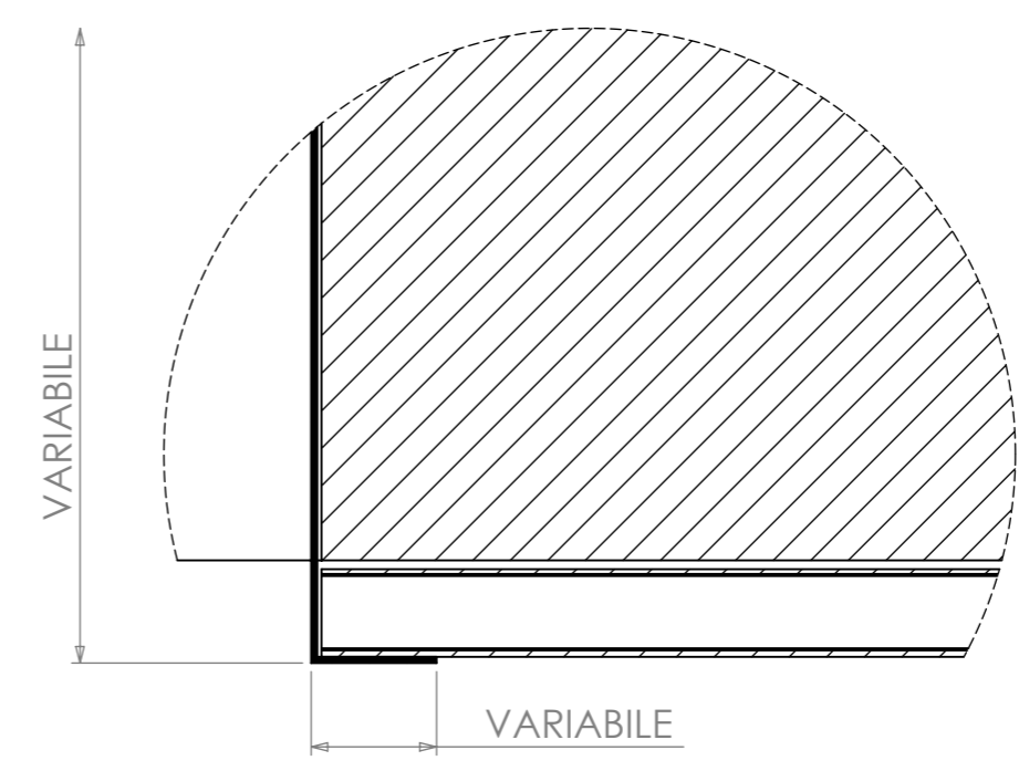
DETTAGLIO E SCALA 1 : 2
